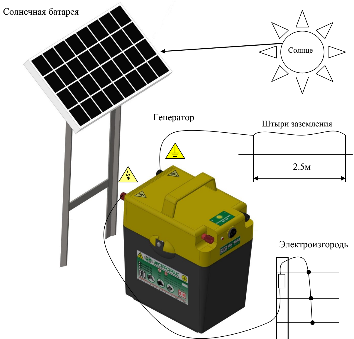
Рисунок 3 - Схема подключения генератора
