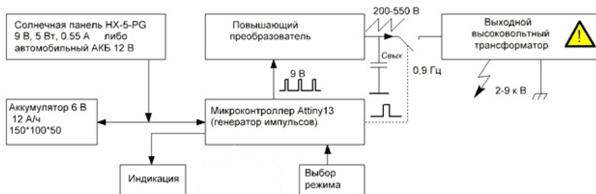
Рисунок 2 - Структурная схема генератора
